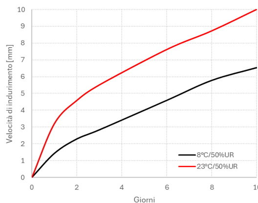
Grafico 1 Velocità di indurimento di POLY-MAR MS 945.
