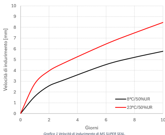
Grafico 1 Velocità di indurimento di MS SUPER SEAL.
