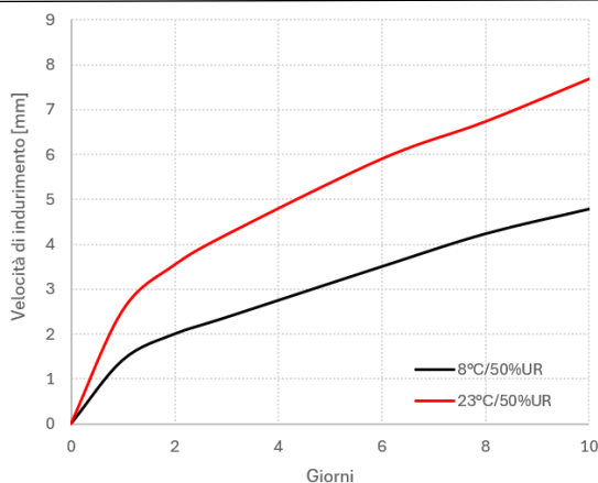
Grafico 1 Velocità di indurimento di MS SPECIAL N.
