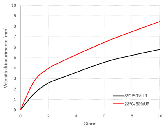
Grafico 1 Velocità di indurimento di MS SHEET VHT.
