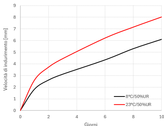
Grafico 1 Velocità di indurimento di MS SUPERFAST.
