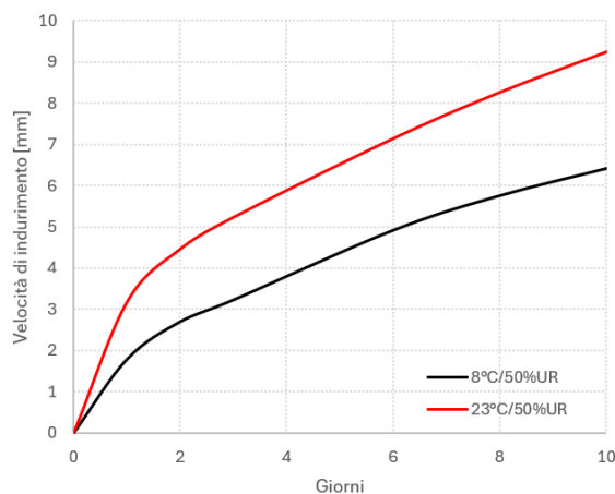
Grafico 1 Velocità di indurimento di MS SUPER.
