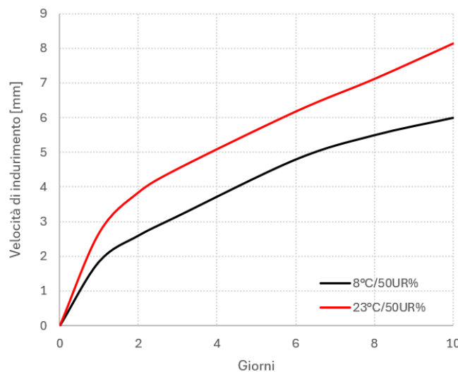
Grafico 1 Velocità di indurimento di MS SCREEN.
