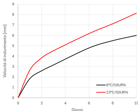
Grafico 1 Velocità di indurimento di MS SCREEN.
